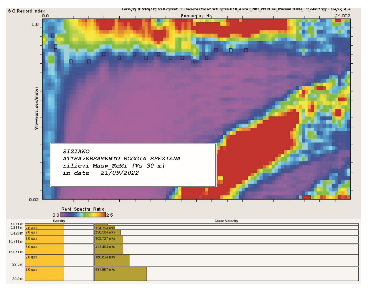
Figura 18 - AREA D'INDAGINE PROFILO 6. Dispersione della velocità di fase delle onde di Rayleigh.
