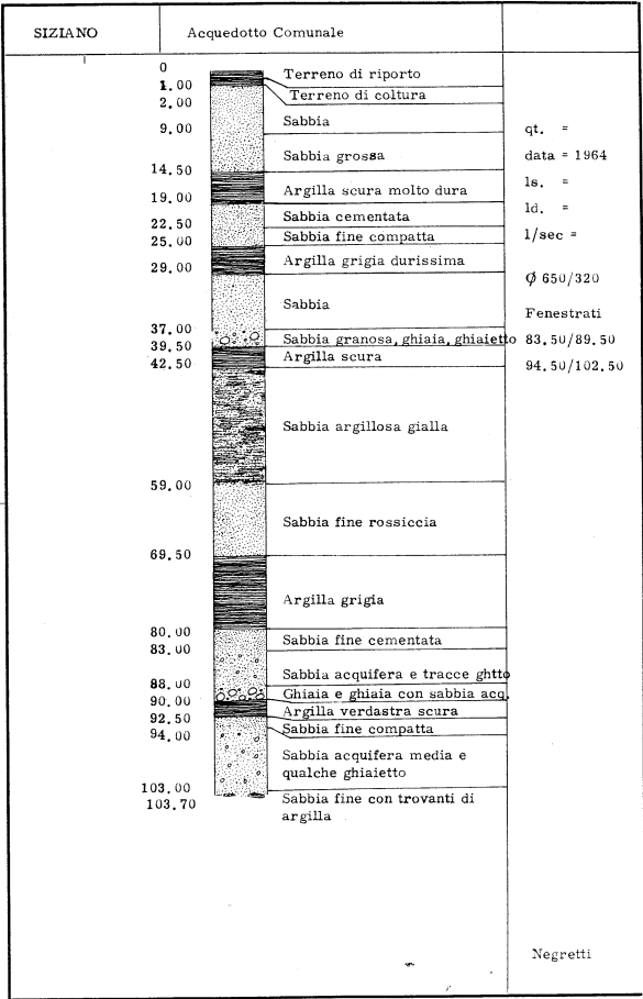
Figura 12 - Stratigrafia di un pozzo ad uso idropotabile del Comune di SIZIANO
