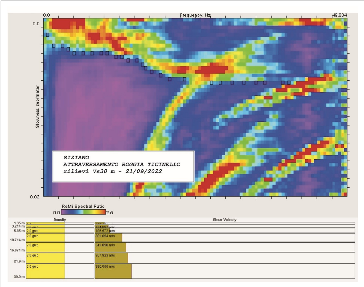
Figura 16 - AREA D'INDAGINE PROFILO 5. Dispersione della velocità di fase delle onde di Rayleigh.
