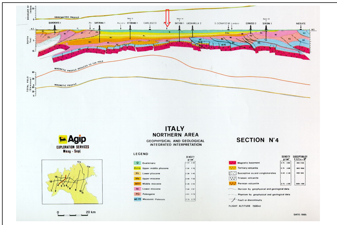
Figura 2 - Struttura del sottosuolo della Pianura Padana nella zona del Comune di SIZIANO. Estratto da: ANELLI-GORZA-GROPPI-RIVA, 1994 – Subsurface well data in the northern Appennines (Italy) – Mem. Soc. Geol. It.
