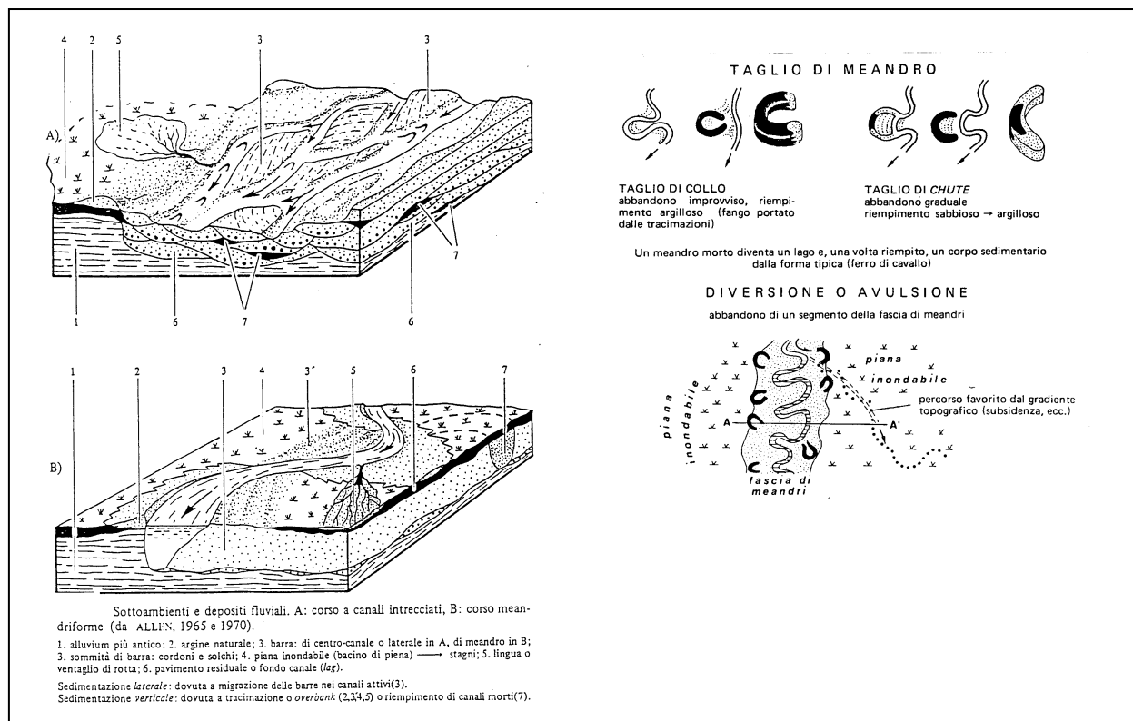
Figura 3 - Sottoambienti e depositi fluviali. A. corso a canali intrecciati. B. corso meandriforme. (ALLEN, 1965 e 1970). Taglio di meandro, diversione o avulsione. (RICCI LUCCHI, 1980).
