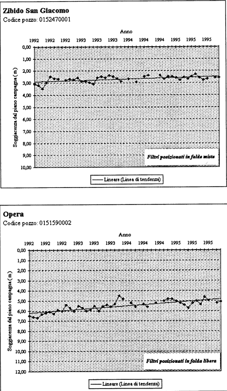
Figura 11 - Escursione pluriennale del livello di soggiacenza della falda freatica superficiale in località limitrofe al territorio di Siziano.
