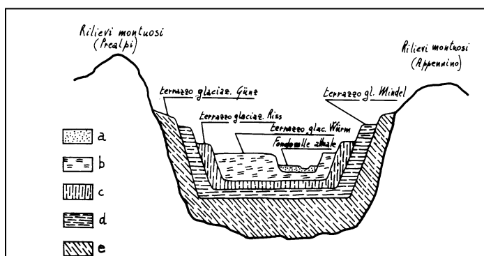
Figura 4 - Rappresentazione schematica della struttura della Pianura padana (A. Pagano). a: alluvioni recenti ed attuali (Olocene); b: Fluviale recente (Würm); c: Fluviale medio (Riss); d: Fluviale antico (Mindel); e: Fluviale basale (Gunz).
