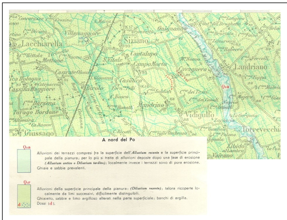
Figura 7 – Carta Geologica d'Italia, F° 59 Pavia, scala 1: 100.000.
