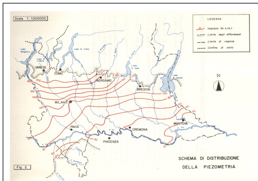
Figura 14 - Morfologia della superficie piezometrica della falda lombarda. Da: Acque da Pozzi. Caratteristiche idrogeologiche principali di alcune zone della pianura lombarda . Regione Lombardia, 1985.
