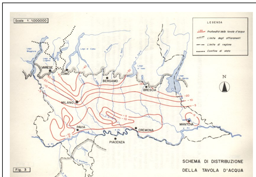
Figura 13 - Morfologia della soggiacenza della falda lombarda. Da: Acque da Pozzi. Caratteristiche idrogeologiche principali di alcune zone della pianura lombarda . Regione Lombardia, 1985.
